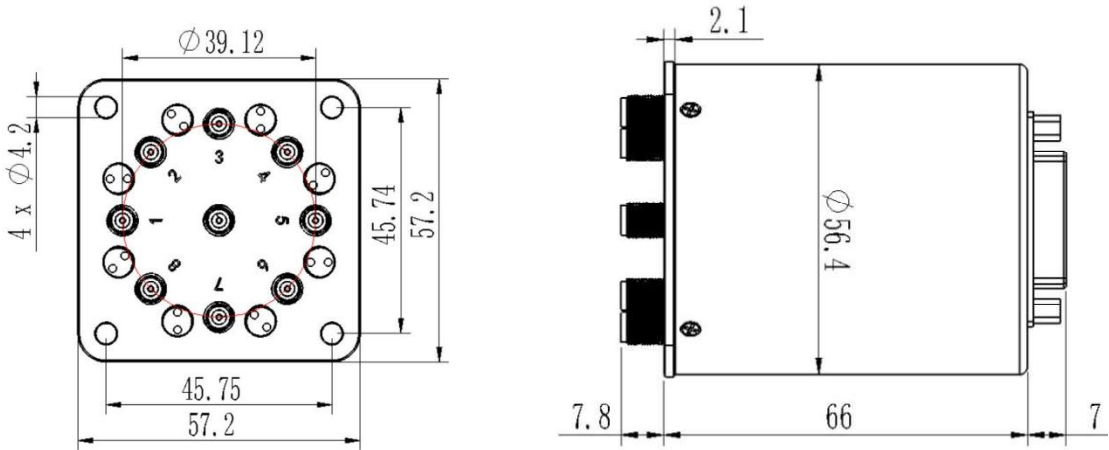
● 俯视图
