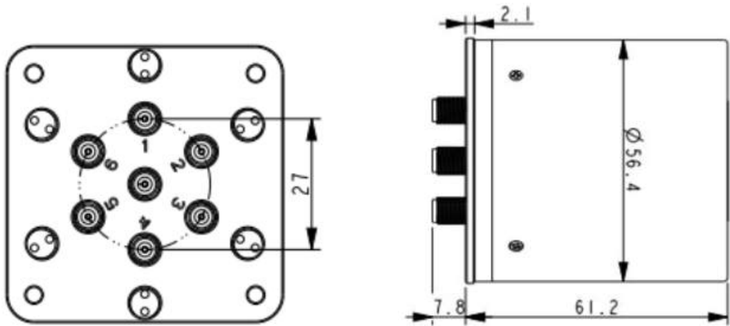
● 俯视图
