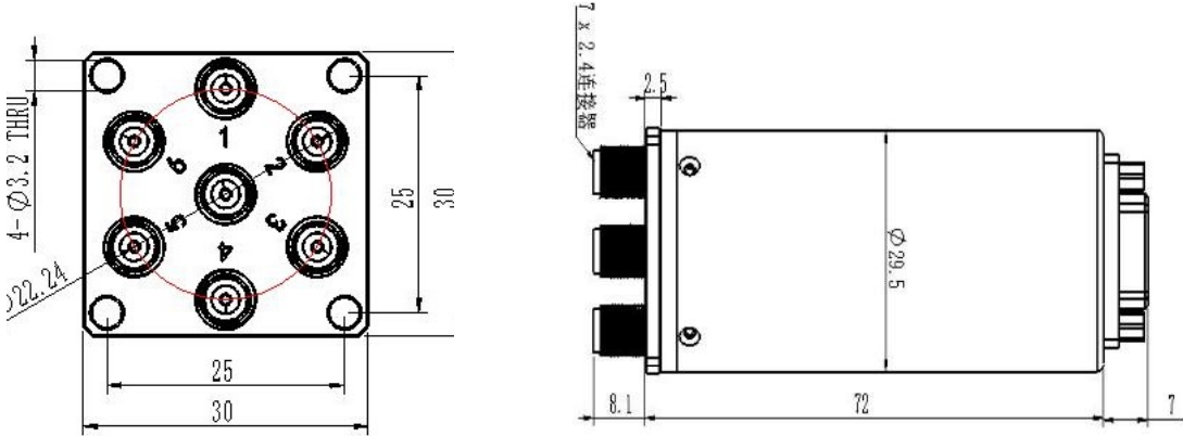
● 俯视图
