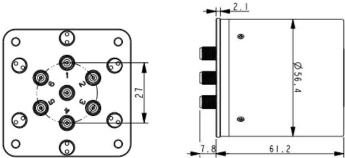
● 俯视图
